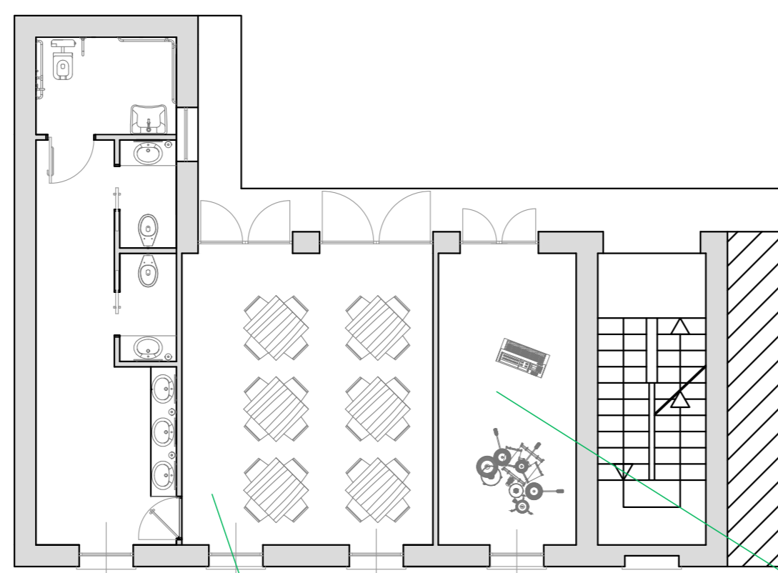
Primo piano
